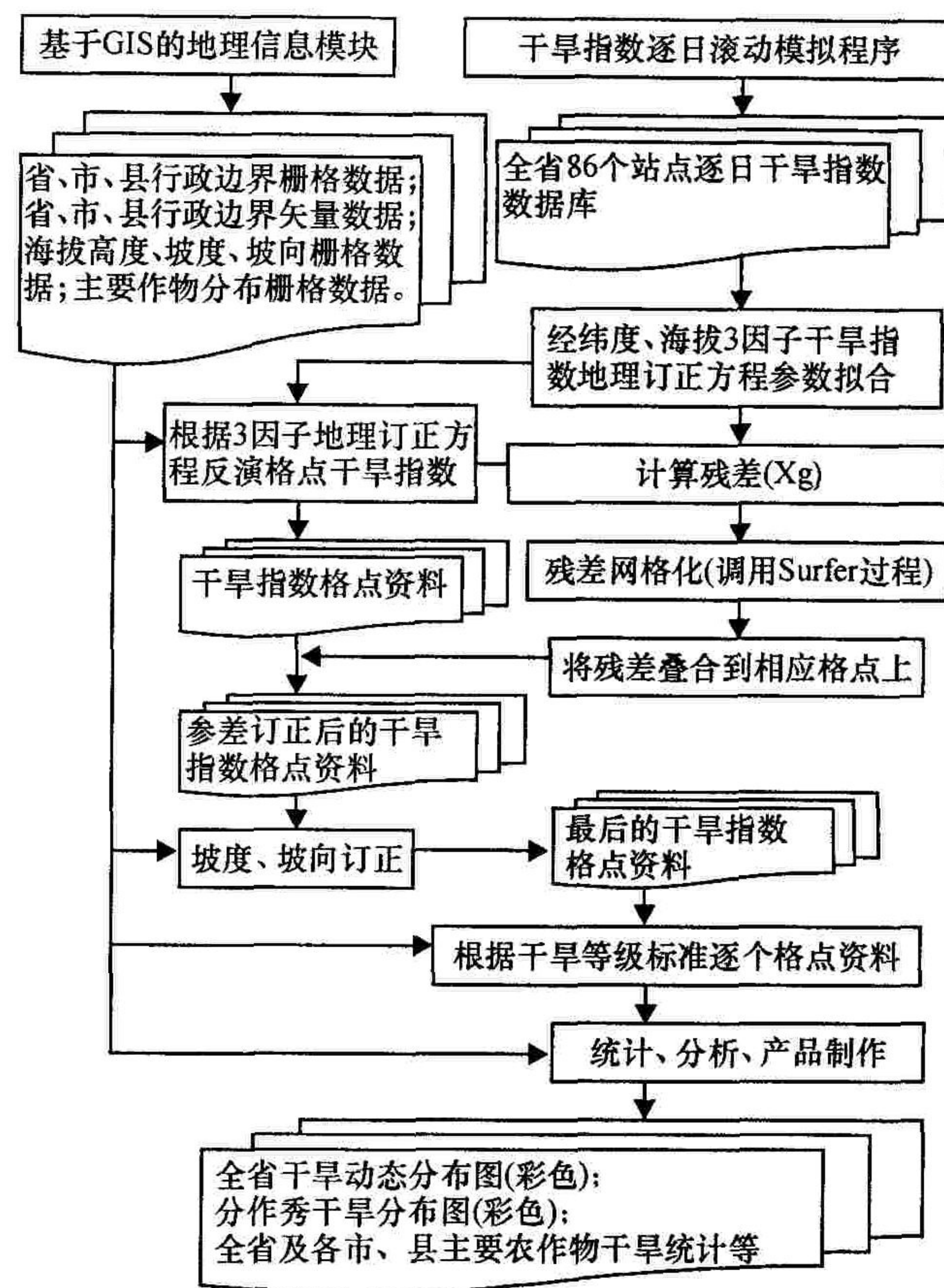
图1 广东省干旱动态监测系统流程图
