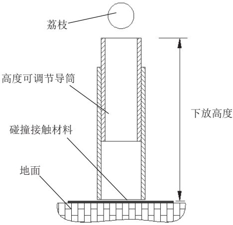
图 1 跌落碰撞试验装置
