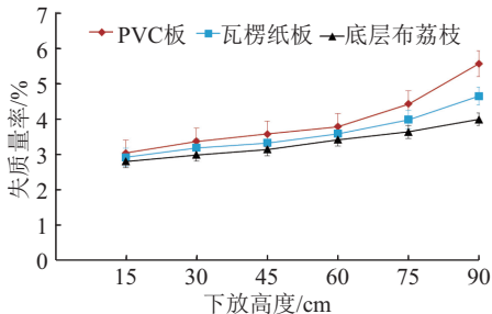
图 4 不同跌落碰撞条件下荔枝失质量率的变化 Fig. 4 Weight loss rate of litchi under different drop collision condition
