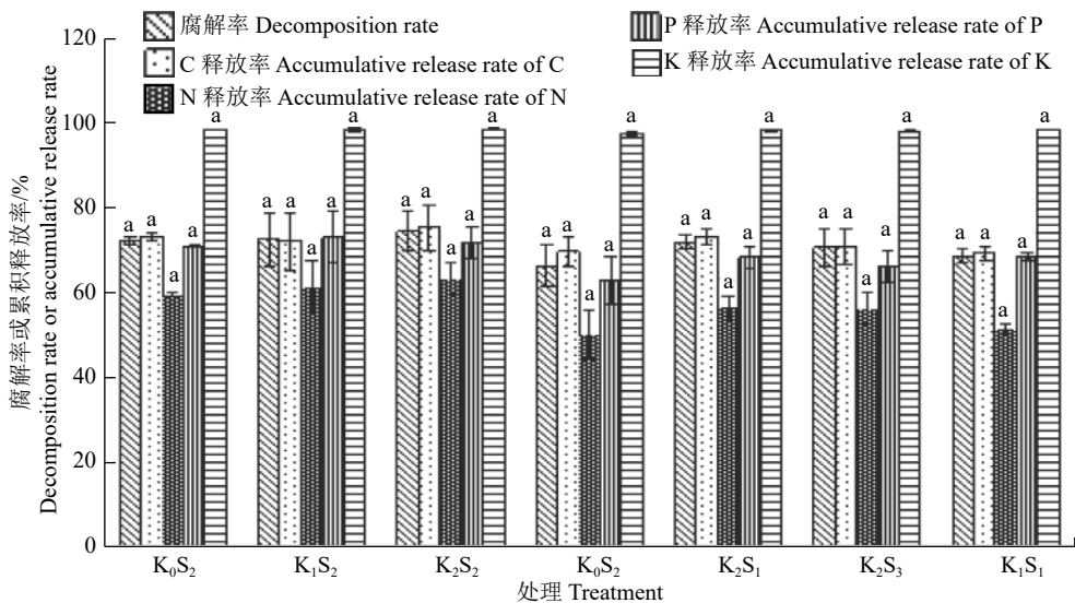
图 2 稻草钾肥配施对稻草腐解率及 C、N、P 和 K 累积释放率的影响
